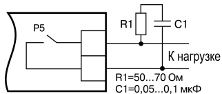
Рисунок 5.3 – Шунтирование контактов реле при работе с индивидуальными нагрузками
