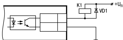
Рисунок 5.4 – Использование транзисторной оптопары для управления реле
