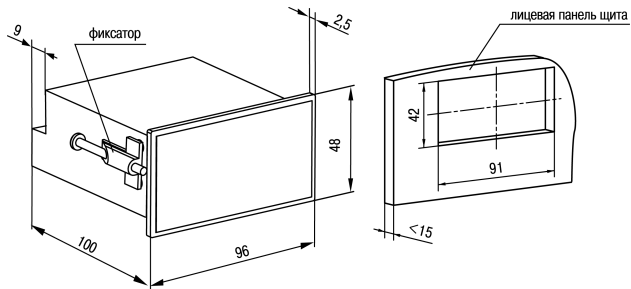
Рисунок 4.2 – Габаритные размеры корпуса Щ2
