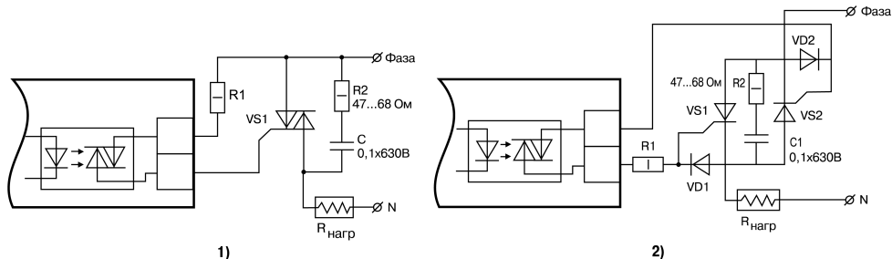
Рисунок 5.5 – Использование симисторной оптопары: 1) для управления силовым симистором, 2) для управления силовыми тиристорами
