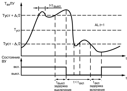
Рисунок 7.3 – Работа ЛУ с задержками включения и выключения
