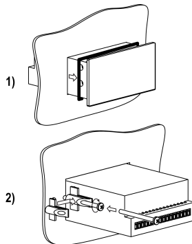
Рисунок 4.1 – Монтаж прибора щитового крепления
