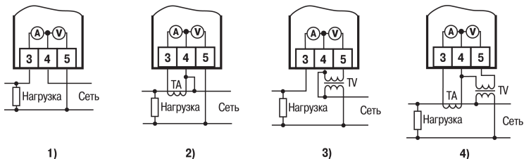
Рисунок 5.2 – Подключение: 1) к однофазной сети, 2) к однофазной сети через согласующий трансформатор тока, 3) к однофазной сети через согласующий трансформатор напряжения, 4) к однофазной сети через согласующие трансформаторы тока и напряжения
