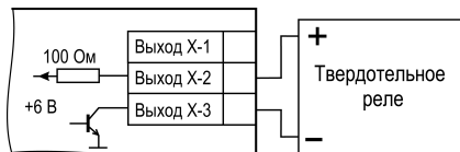
Рисунок 5.6 – Схема подключения к ВУ типа Т
