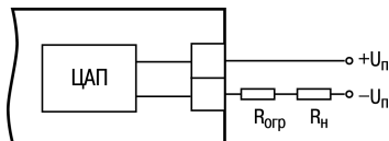
Рисунок 5.7 – Схема соединения ЦАП с нагрузкой
