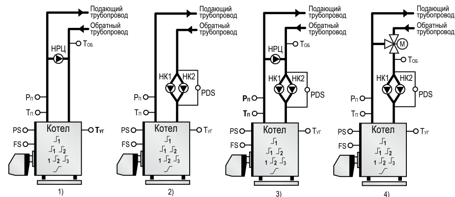
Рисунок 1.1 – Объект управления
