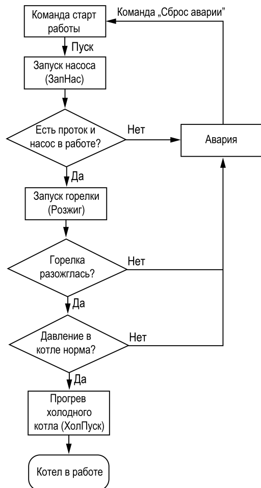
Рисунок 10.1 – Алгоритм запуска
