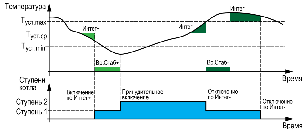
Рисунок 10.2 – Регулирование температуры
