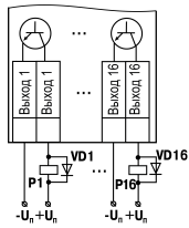
Рисунок 9 – Схема подключения нагрузок к ВЭ типа «К»
