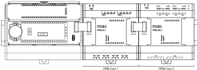
Рисунок 14 – Расположение модулей расширения на шине
