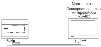
Рисунок 10 – Типовая схема подключения в режиме Slave
