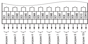
Рисунок 4 – Схема подключения нагрузок к ВЭ типа «Р»
