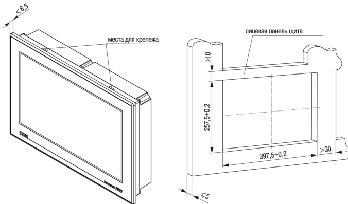
Рисунок 3 – Установочные размеры СП315
