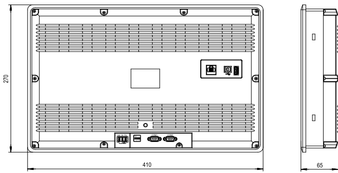
Рисунок 2 – Габаритные размеры СП315
