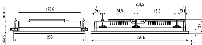
Рисунок 3 – Дополнительные установочные размеры прибора
