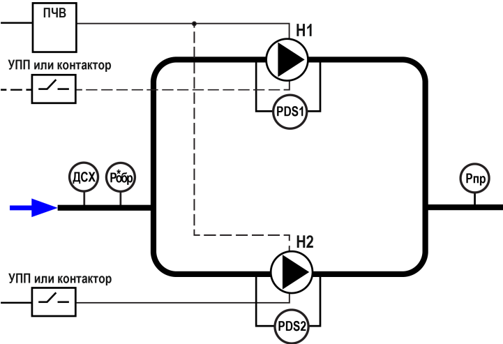
Рисунок 4 – Объект управления
