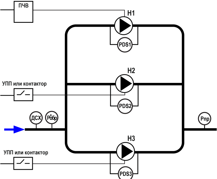
Рисунок 4 – Объект управления
