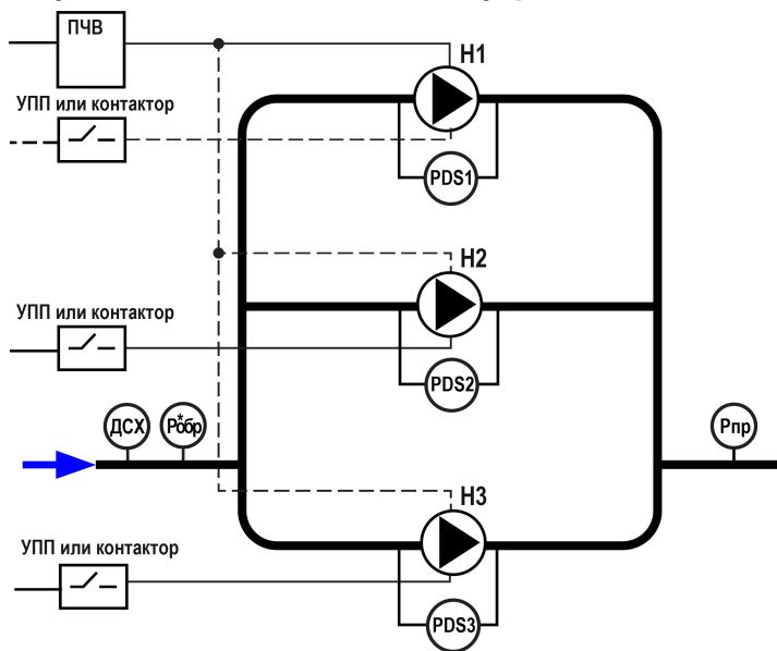
Рисунок 4 – Объект управления
