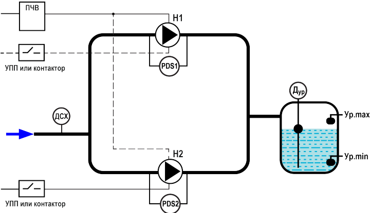
Рисунок 4 – Объект управления
