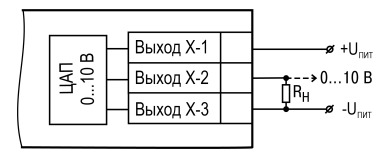
Рисунок 10 – Схема подключения нагрузки к ВУ типа «У»
