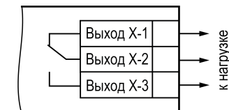
Рисунок 9 – Подключение нагрузки к ВУ типа «Р»
