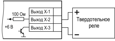
Рисунок 11 – Подключение нагрузки к ВУ типа «Т»
