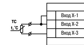
Рисунок 5 – Двухпроводная схема подключения ТС
