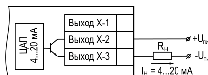
Рисунок 5.23 – Подключение к ВУ типа «И»
