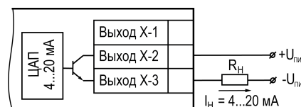
Рисунок 5.24 – Подключение к ВУ типа «И»
