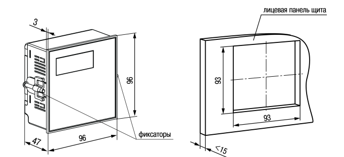
Рисунок 6 – Габаритные размеры корпуса Щ11
