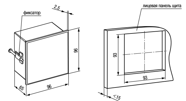
Рисунок 2 – Габаритные размеры корпуса Щ1
