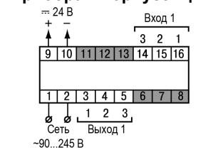
Рисунок 12 – Назначение контактов клеммной колодки прибора в DIN-реечном Д корпусе
