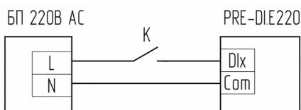
Е - «сухой контакт» с внешним питанием 220В
