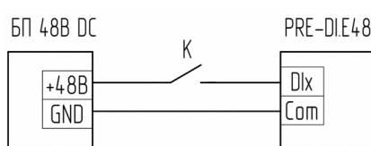
Е - «сухой контакт» с внешним питанием 48В
