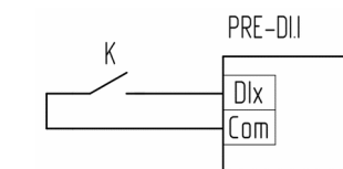
І - «сухой контакт» без внешнего питания
