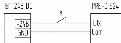
Е - «сухой контакт» с внешним питанием 24В
