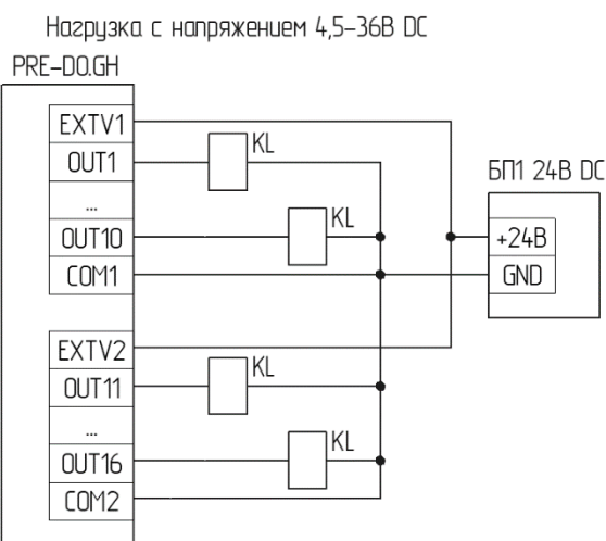
Рис. П1.4 Внешний вид и схема подключения модулей серии PRE-16DO.GH-RS24
