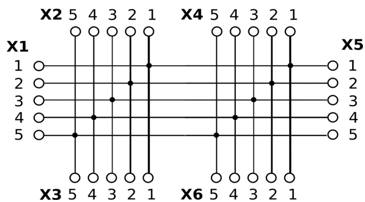
Принципиальная схема
