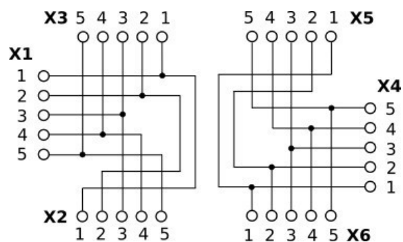
Рис. 1. Схема принципиальная ПР-6Д
