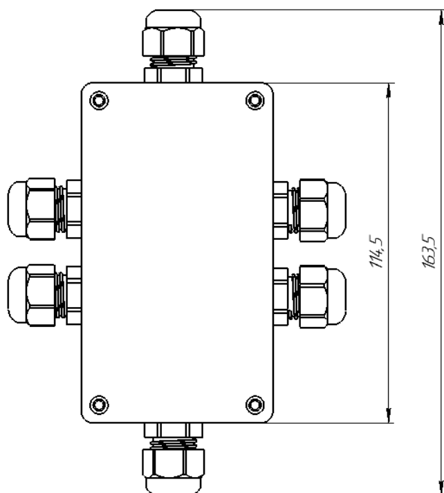
Рис. 2. Габаритные и установочные размеры ПР-6Д IP65
