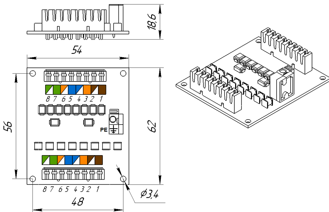
Рис. 1. Размеры и внешний вид
