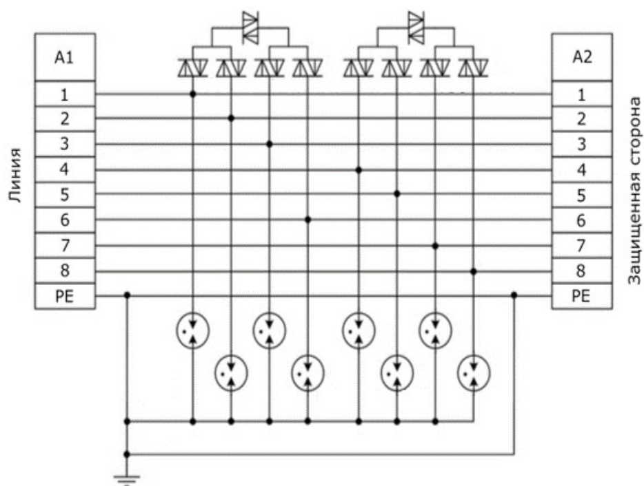
Рис. 2. Принципиальная схема
