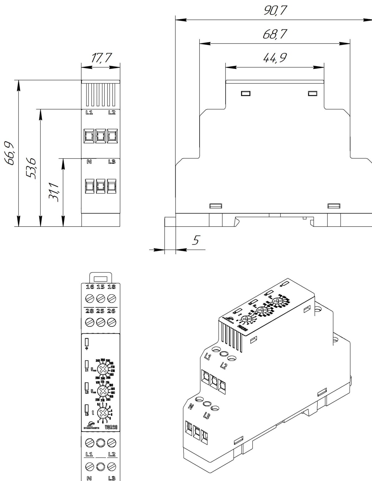
Рис. 4. Габаритные размеры реле контроля напряжения VCR20
