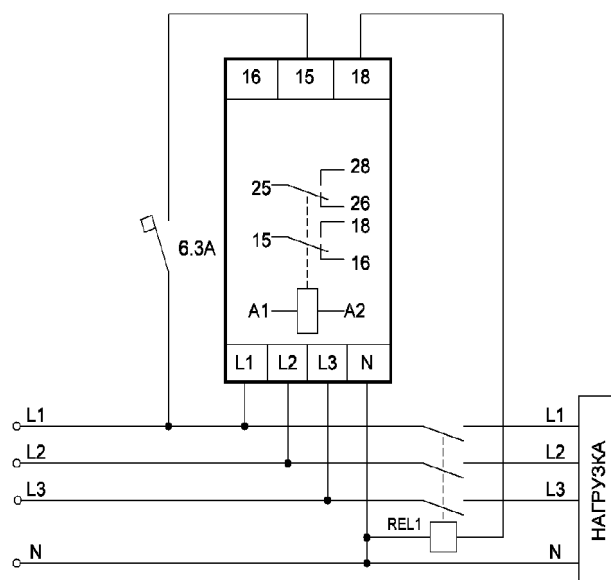
Рис.1 Принципиальная схема подключения реле контроля напряжения VCR20
