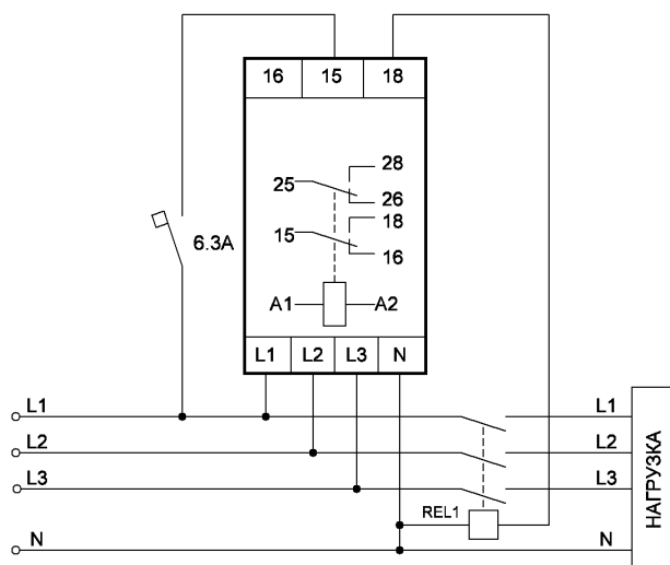
Рис.1 Принципиальная схема подключения реле контроля напряжения VCR21
