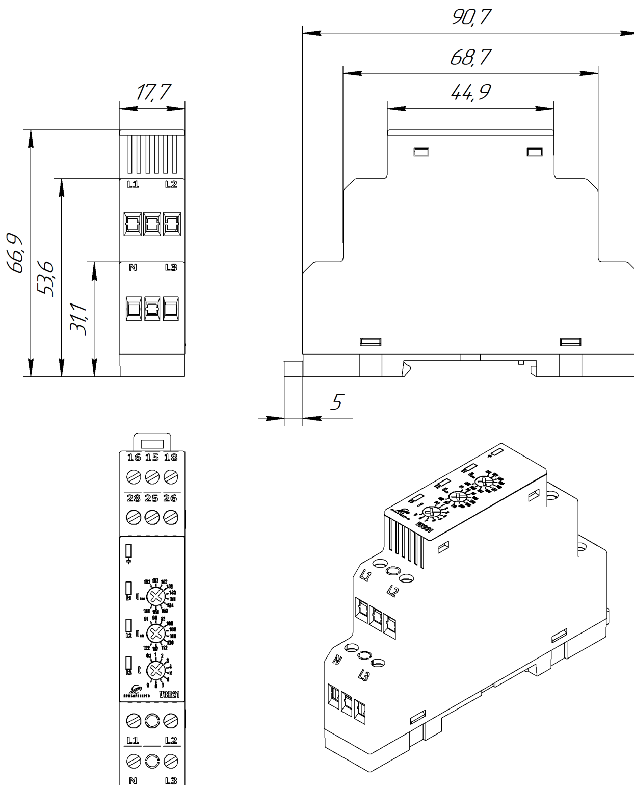
Рис. 4. Габаритные размеры реле контроля напряжения VCR21
