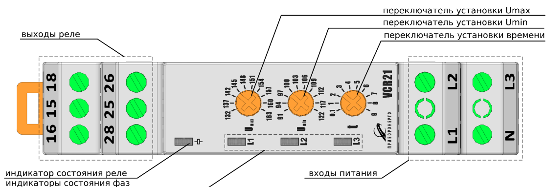
Рис.2 Панель управления и индикации реле контроля напряжения VCR21
