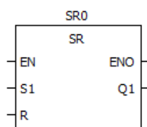
Рисунок 5.5 – Изображение элементарного функционального блока с параметрами EN/ENO
