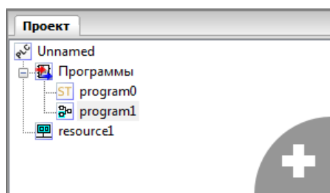
Рисунок 151 – Проект, содержащий два программными модулями типа «Программа»
