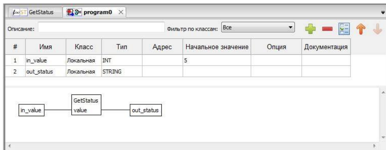
Рисунок 138 – Пример FBD диаграммы с использованием пользовательской функции
