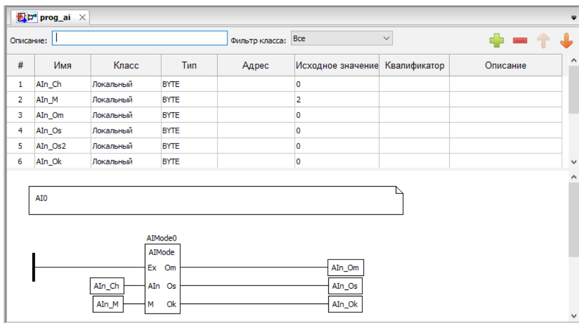
Рисунок 13 – Редактор программы с панелью констант и переменных
