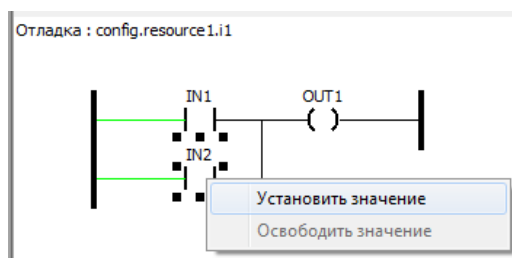
Рисунок 179 – Пример отладки LD диаграммы
