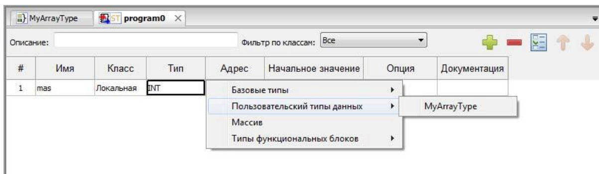
Рисунок 158 – Выбор добавленного типа данных в панели переменных и констант программного модуля
