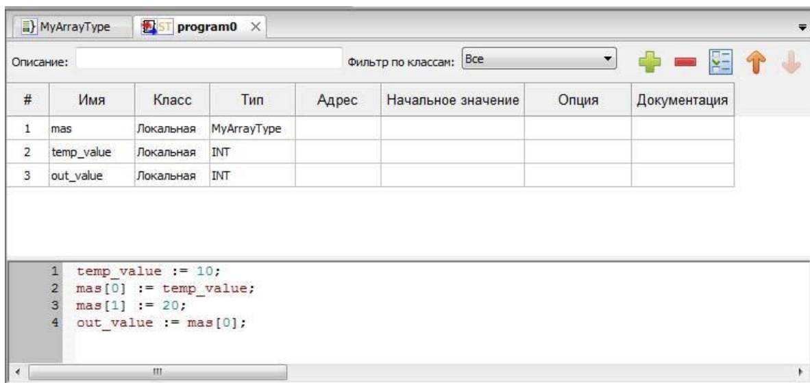
Рисунок 159 – Пример использования массива в коде на языке ST
