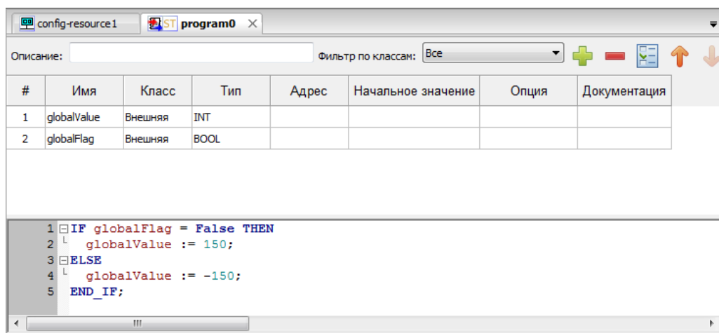
Рисунок 145 – Объявление и использование глобальных переменных ресурса
