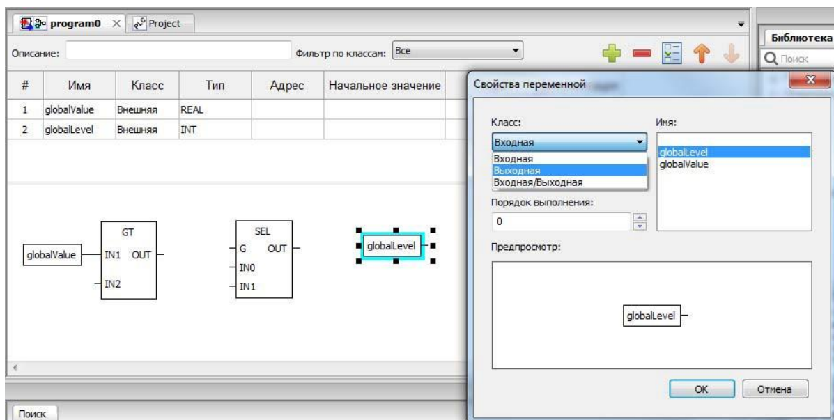
Рисунок 125 – Указание класса «Выходная» для переменной
