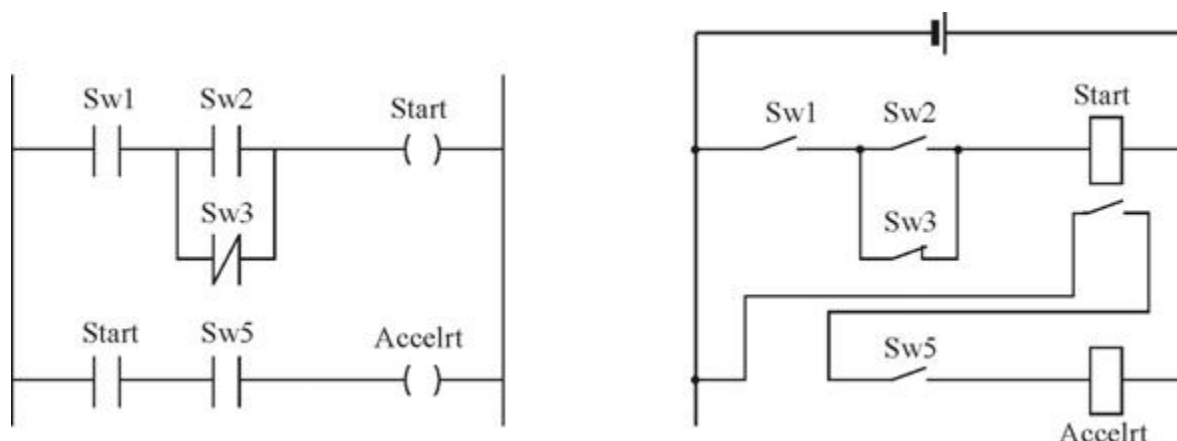
Рисунок 6.1 – Программа на языке LD (слева) и ее эквивалент в виде электрической (справа)
