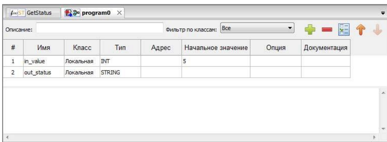
Рисунок 134 – Добавленный программный модуль «Программа» на языке FBD
