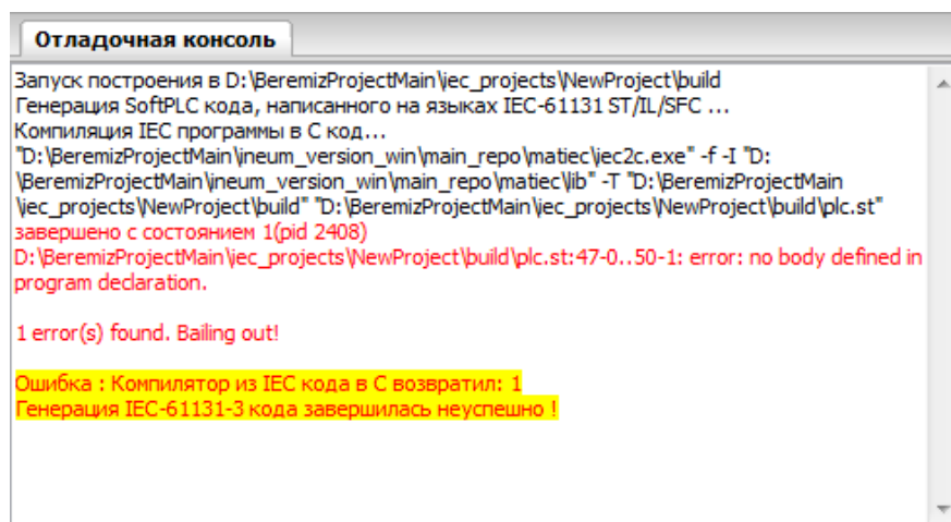
Рисунок 97 – Ошибка сборки проекта в отладочной консоли
