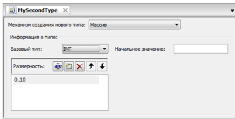
Рисунок 88 – Добавление типа данных «Массив»
