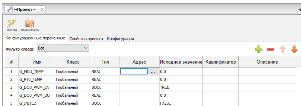
Рисунок 104 – Поле «Адрес» панели переменных и констант
