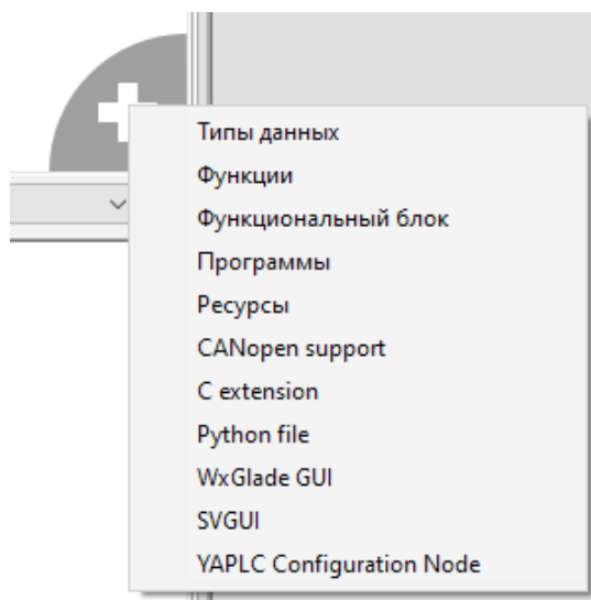
Рисунок 6 – Меню выбора добавляемого элемента в дерево проекта
