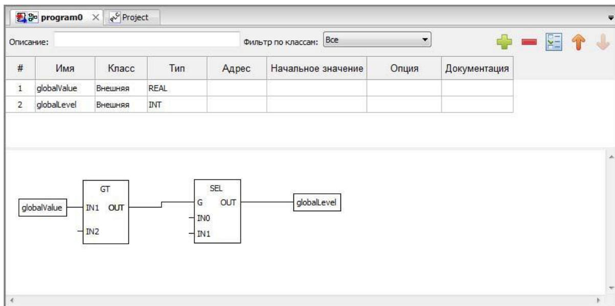
Рисунок 126 – Соединение входов и выходов функций на диаграмме FBD
