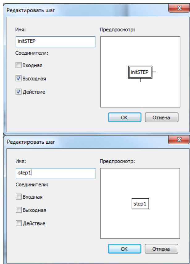
Рисунок 55 – Диалоги редактирования шага инициализации и обычного шага SFC диаграммы
