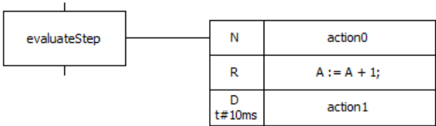
Рисунок 7.6 – Шаг «evaluateStep» и связанный с ним блок действий, содержащий 3 действия
