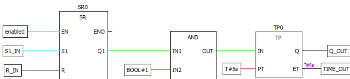
Рисунок 5.10 – Выполнение FBD диаграммы
