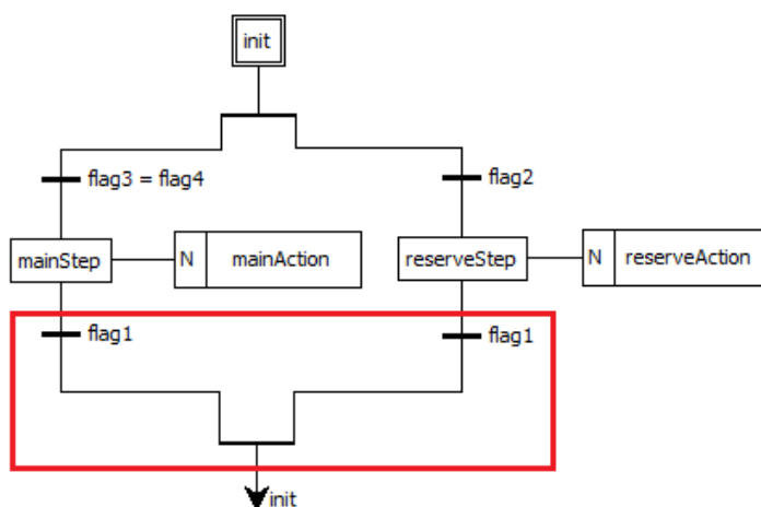
Рисунок 73 – Пример SFC диаграммы, содержащей конвергенцию
