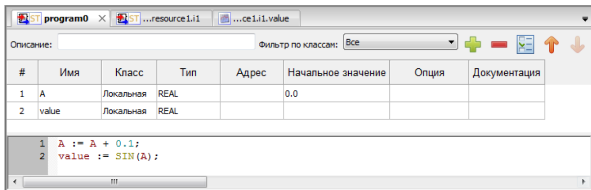
Рисунок 187 – Пример программного модуля тип «Программа» на языке ST
