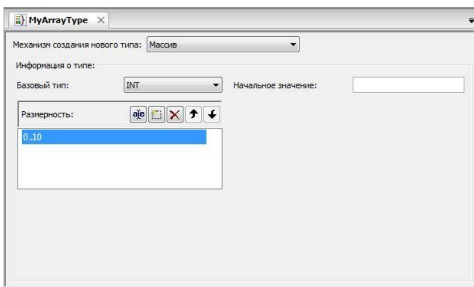
Рисунок 157 – Задание размерности для массива
