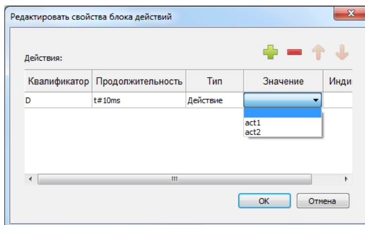
Рисунок 67 – Выбор предопределённого действия
