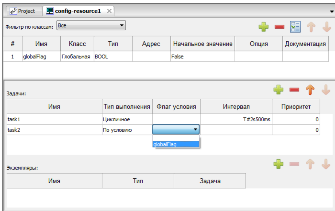
Рисунок 150 – Выбор переменной типа BOOL для определения условия выполнения задачи
