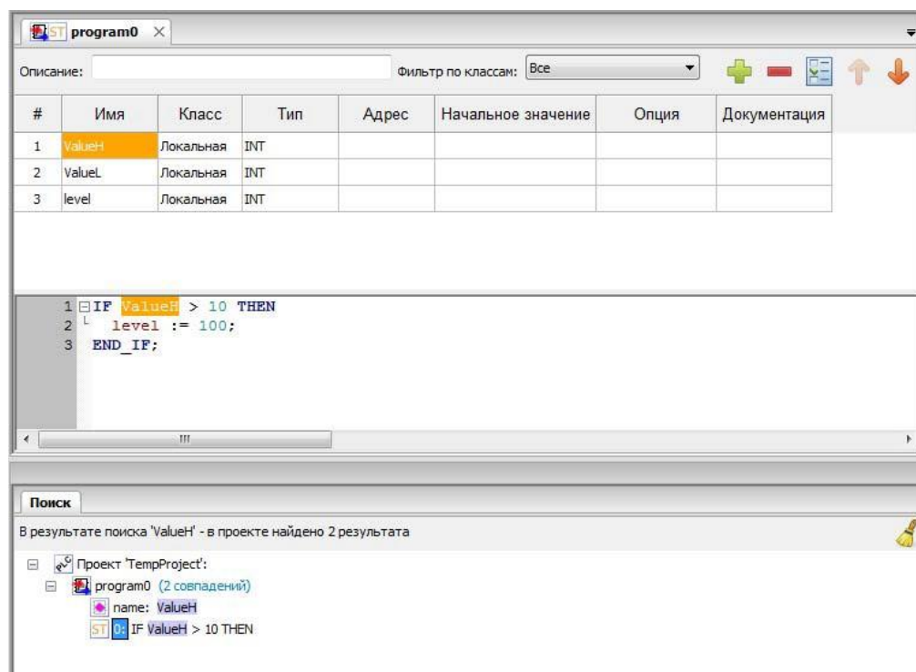
Рисунок 99 – Результат примера поиска элемента в проекте
