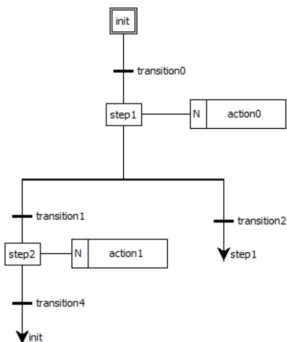
Рисунок 7.7 – SFC диаграмма, содержащая «прыжки»
