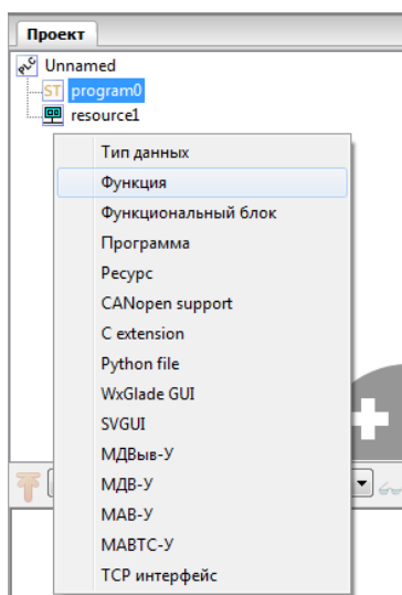
Рисунок 130 – Выбор в дереве проекта добавления функции
