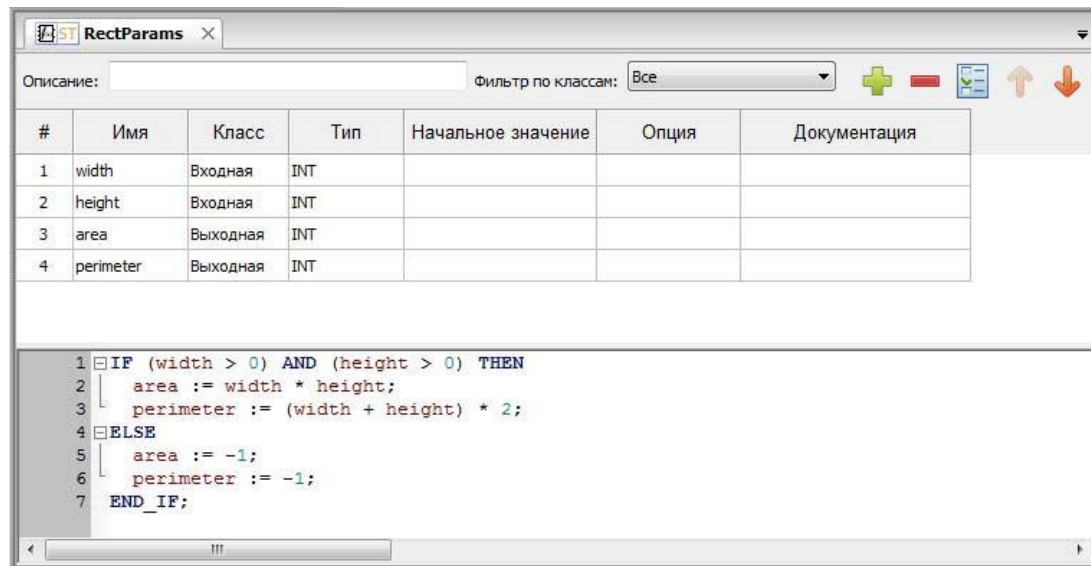
Рисунок 140 – Описание пользовательского функционального блока на языке ST
