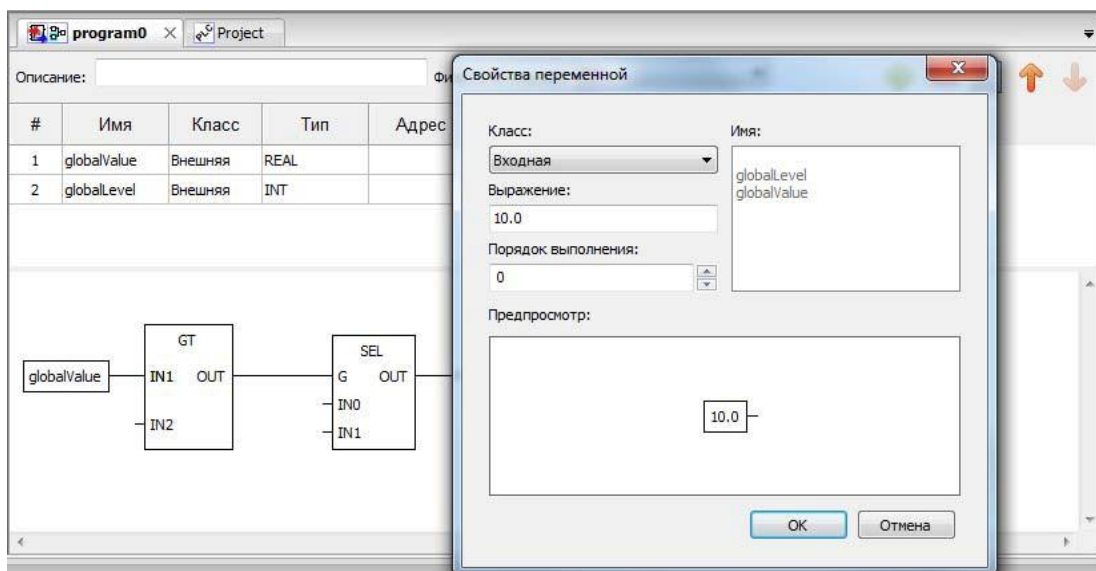
Рисунок 127 – Добавление переменной на FBD диаграмму
