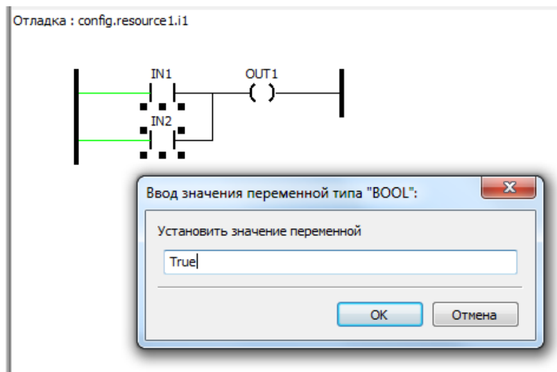
Рисунок 180 – Отладка LD диаграммы
