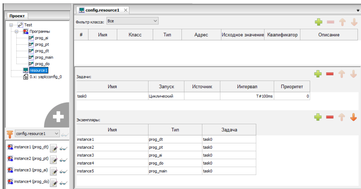
Рисунок 83 – Вкладка ресурс главной рабочей области
