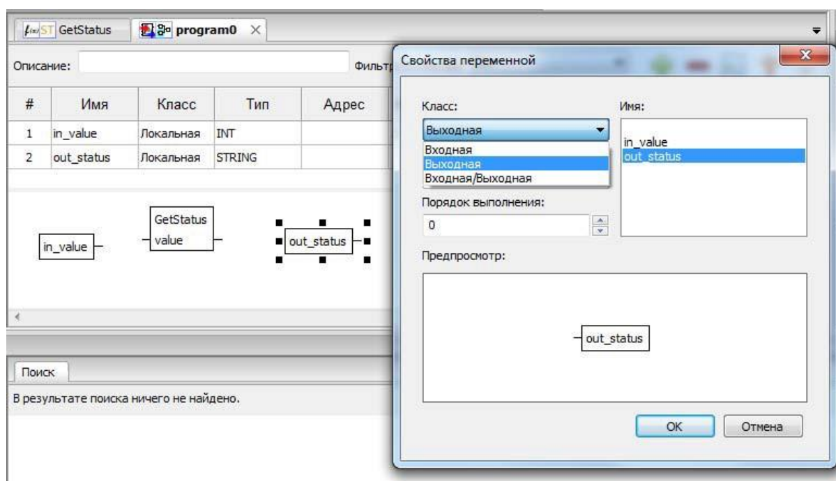
Рисунок 137 – Изменение «класса» переменной FBD диаграммы
