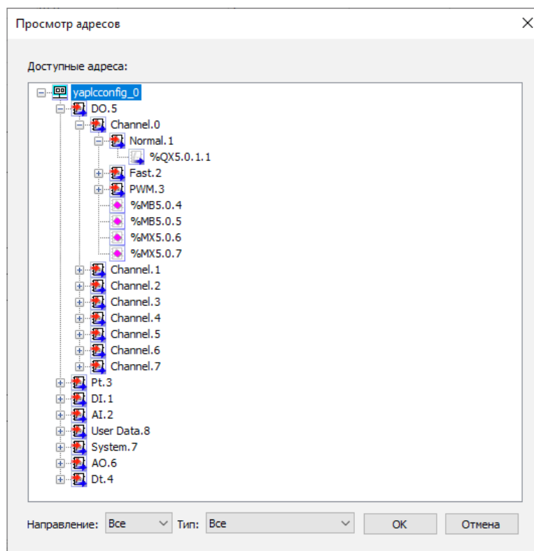
Рисунок 18 – Диалог просмотра адресов регистров УСО
