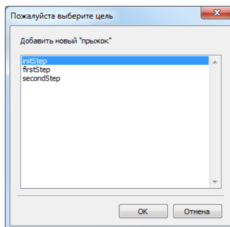
Рисунок 75 – Диалог добавления «прыжка»
