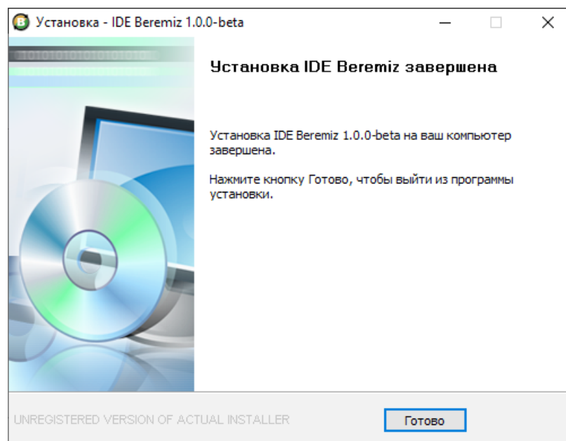
Рисунок 1.5 – Подтверждение установки
