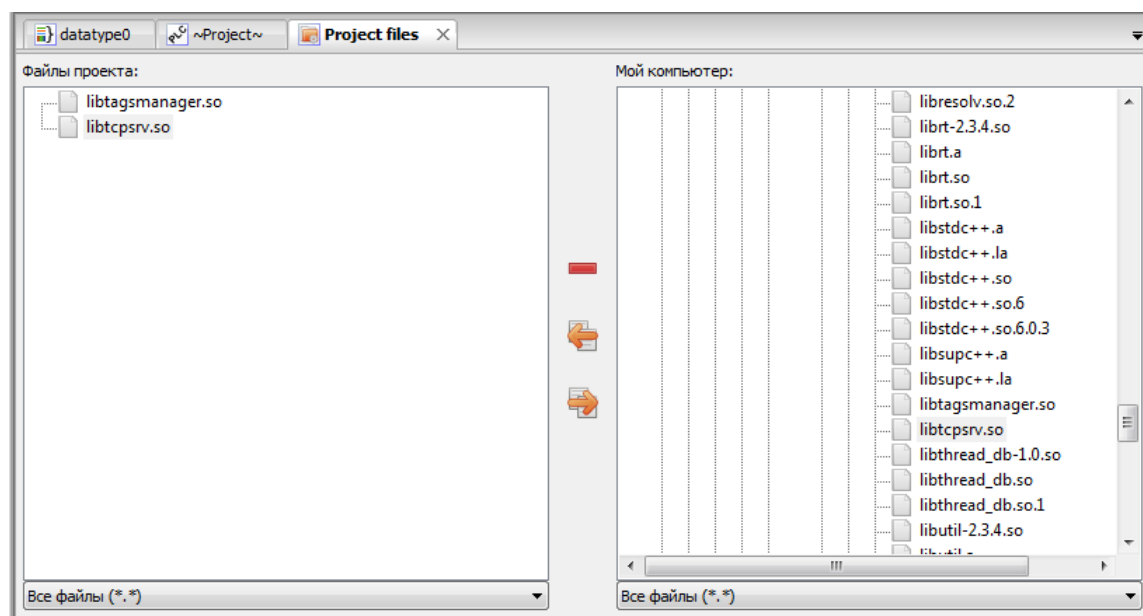
Рисунок 31 – Встроенный проводник
