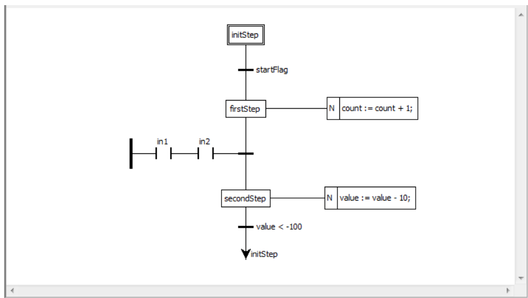
Рисунок 7.12 – SFC диаграмма
