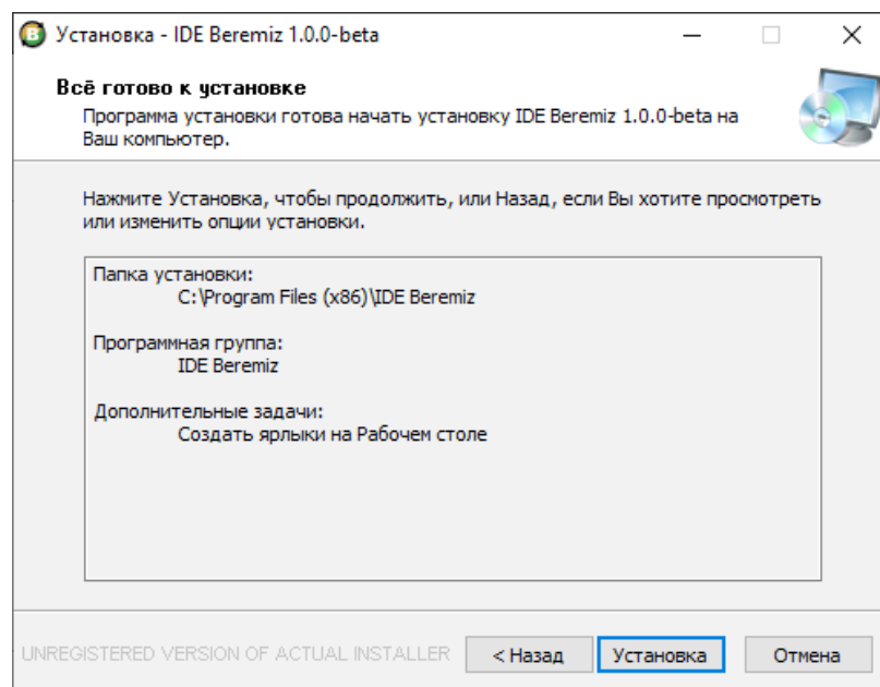
Рисунок 1.4 – Подтверждение установки
