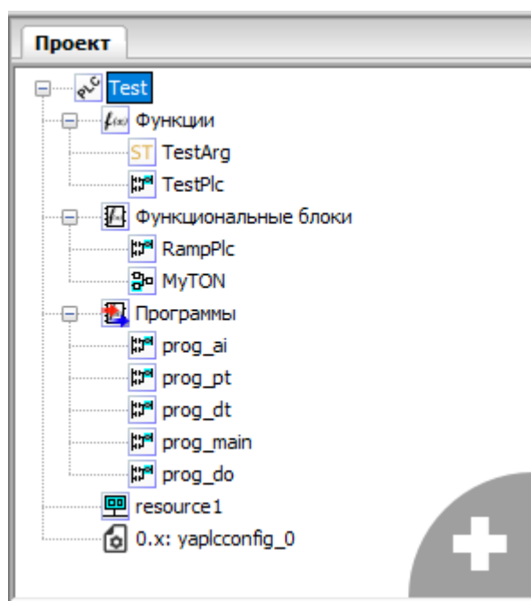
Рисунок 5 – Дерево проекта
