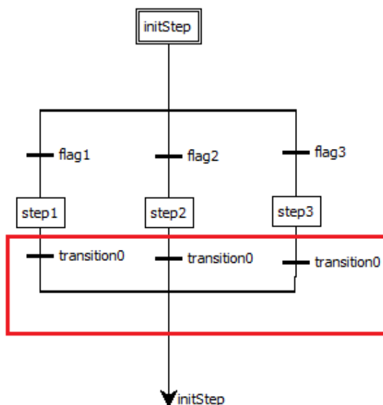
Рисунок 7.9 – Конвергенция на SFC диаграмме
