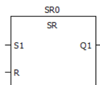
Рисунок 5.3 – Изображение функционального блока в языке FBD
