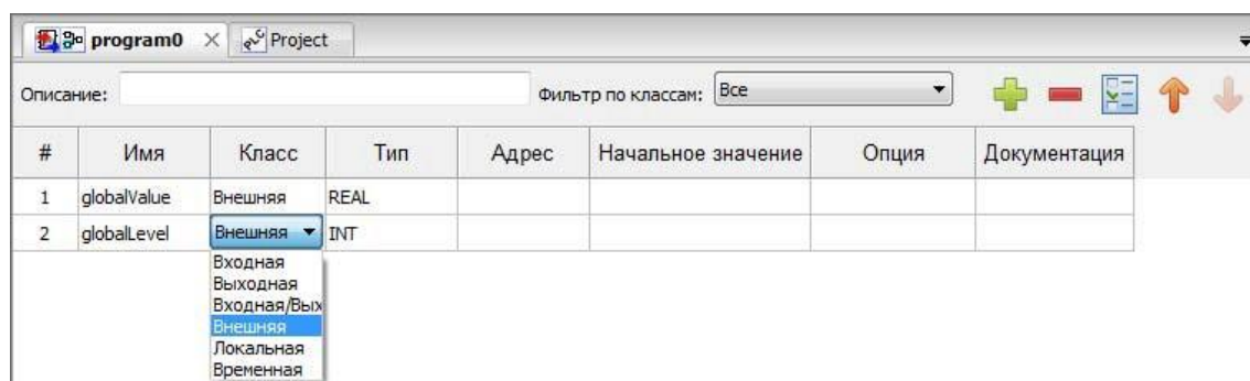
Рисунок 121 – Объявление в программе внешних переменных
