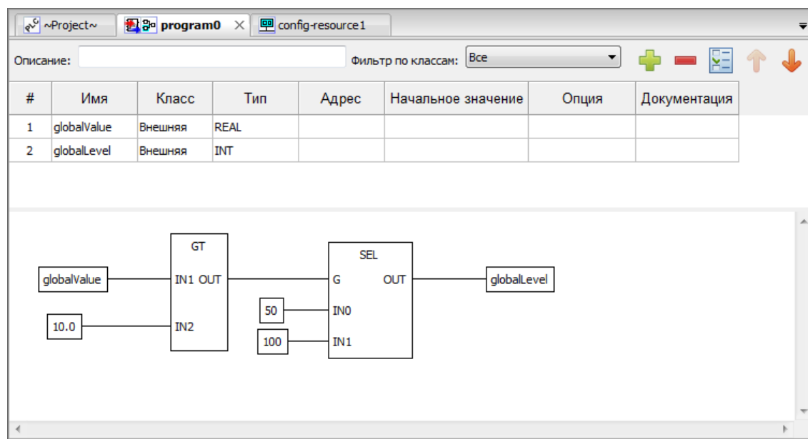
Рисунок 129 – Пример программного модуля, написанного на языке FBD
