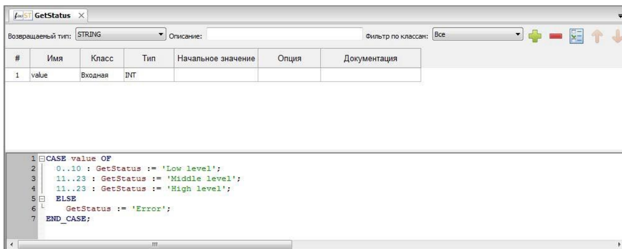
Рисунок 133 – Определение функции алгоритма и логики выполнения
