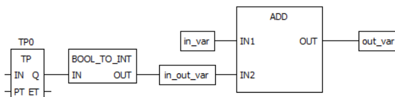
Рисунок 5.4 – Пример соединения переменных, функций и функциональных блоков
