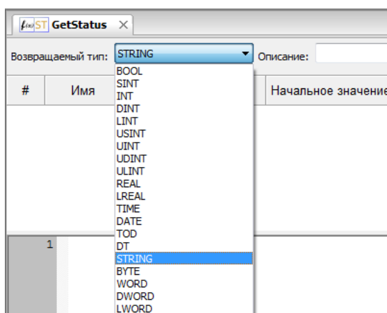
Рисунок 132 – Выбор значения, возвращаемого функцией
