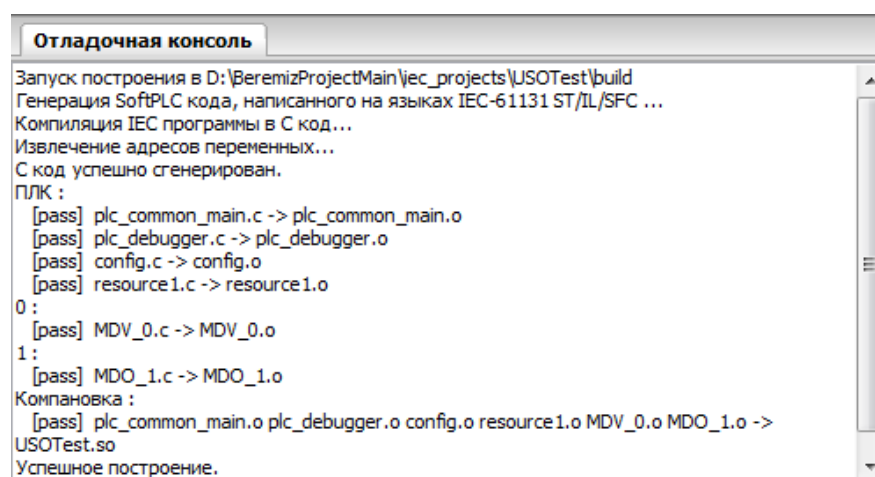
Рисунок 96 – Успешная сборка в отладочной консоли
