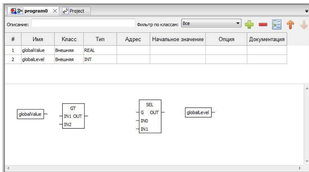
Рисунок 124 – Перенесённые переменные на FBD диаграмму
