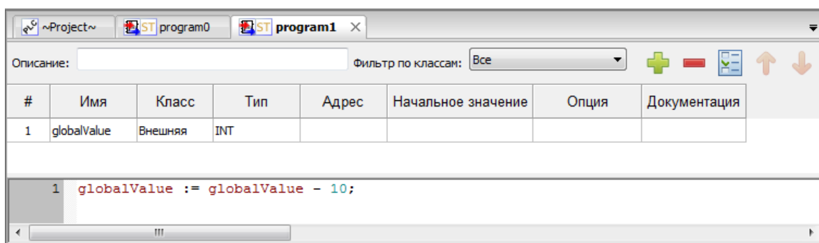
Рисунок 114 – Использование глобальной переменной в программном модуле «program1»
