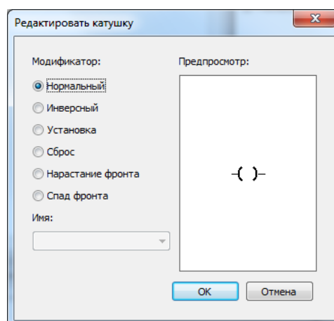
Рисунок 51 – Редактирование катушки
