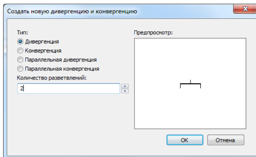
Рисунок 71 – Добавление дивергенции
