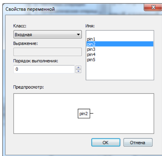
Рисунок 37 – Свойства переменной
