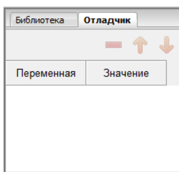
Рисунок 100 – Панель отладки
