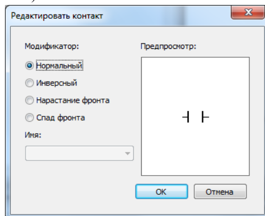
Рисунок 49 – Редактирование контакта
