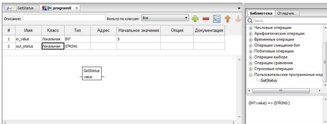
Рисунок 135 – Добавление на FBD диаграмму пользовательской функции
