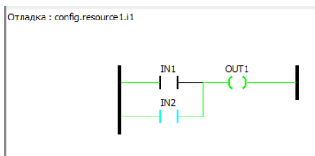
Рисунок 181 – Отладка LD диаграммы
