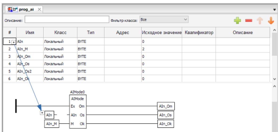
Рисунок 36 – Добавление переменной из панели переменных и констант
