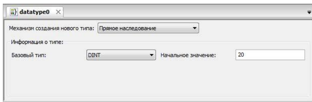
Рисунок 85 – Добавление псевдонима типа данных
