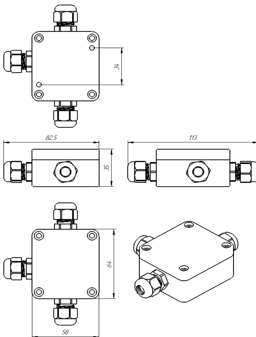
Рисунок А.1 – Габаритные и установочные размеры ПР-3
