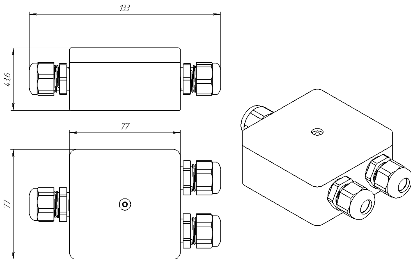
Рисунок А.1 – Габаритные и установочные размеры ПР-3У
