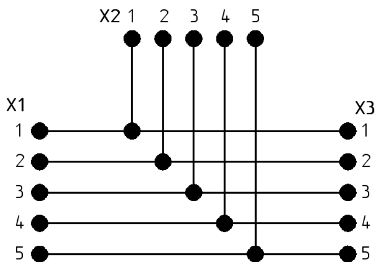
Рисунок А.2 – Схема принципиальная ПР-3У
