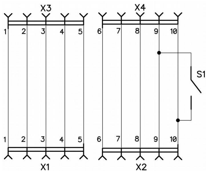
Рисунок А.2 – Схема принципиальная ПР-3Д ТМП КИР
