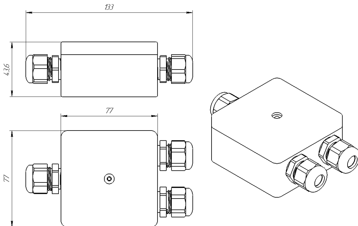
Рисунок А.1 – Габаритные и установочные размеры ПР-3Д ТМП КИР
