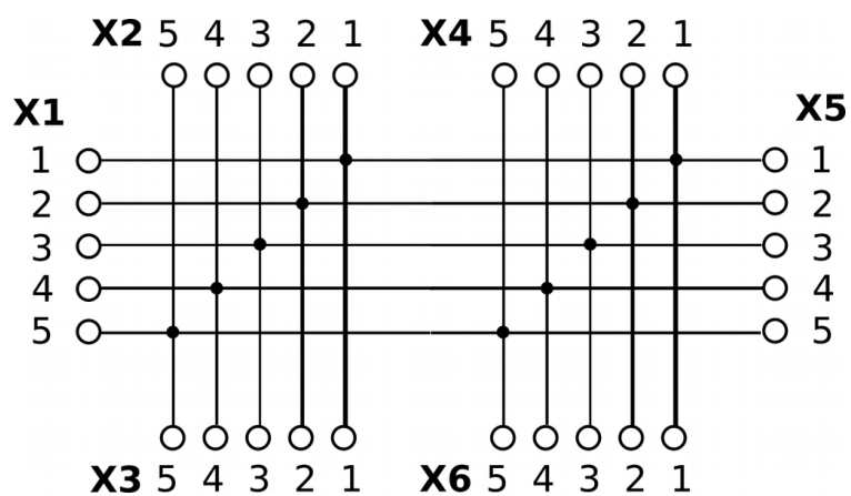
Рисунок А.2 – Схема принципиальная ПР-6 DIN
